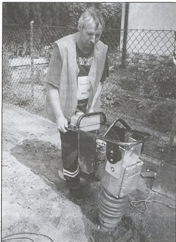
Zagęszczanie ziemi
