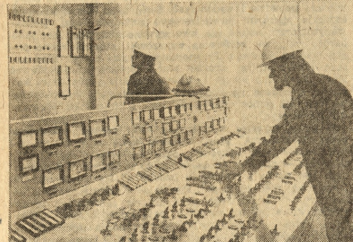
Coraz bardziej skomplikowane jest sterowanie urządzeniami energetycznymi. Na zdjęciu: w nastawni bloku elektrociepłowni „Karolin”.
