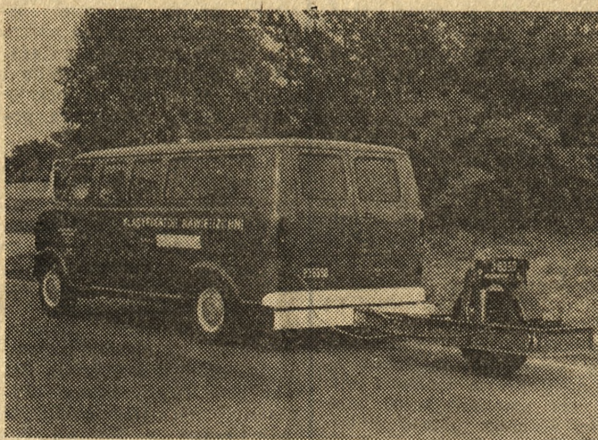
Specjalne urządzenie używane do pomiaru równości nawierzchni drogi.
