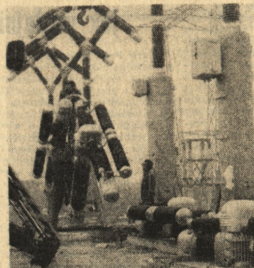
Na zdjęciu: trwa tym elementem naszego krajoobrazu stały się linie przesyłowe energii elektrycznej. Przybywa ich z każdym rokiem. Tak wygląda montaż wyłączników w rozdzielni 400 kV.
