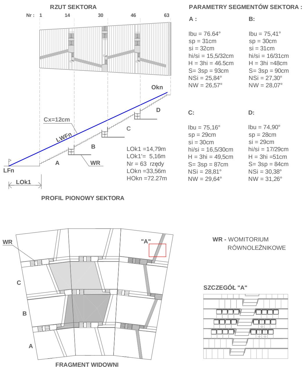
RYŚ. 5-14 PRZYKŁADOWA WIDOWNIA Z ZASTOSOWANIEM SCHODÓW UKOŚNYCH, NAPRZEMIEN- NEGÓ UKŁADU SIEDZISK I WOMITORIÓW RÓWNOLEŻNIKOWYCH.
