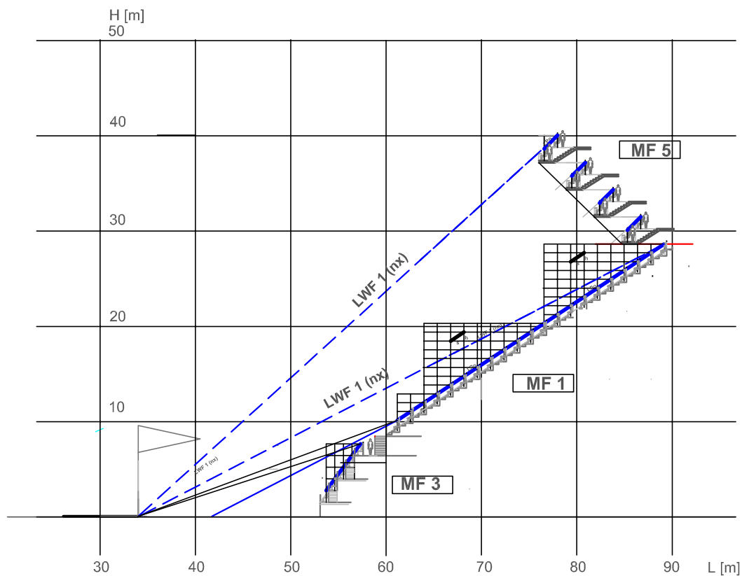
RYS. 5-24 MODEL PROFILU STROMEGO MPS 1 (Złożenie modułów MF 3, MF 1 i MF 5)
