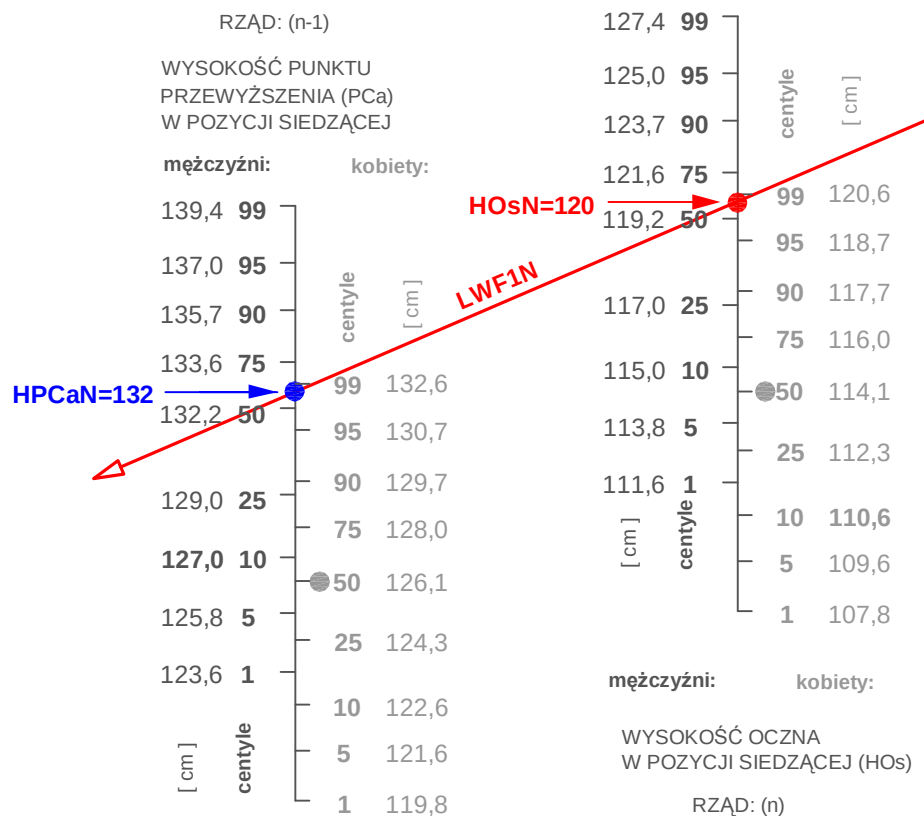
RYS. 2-41 WYKRES POŁOŻENIA LINII WIDZENIA FOKUSÓW BLIŻSZYCH DLA NORMATYWNEJ WYSOKOŚCI OCZNEJ W POZYCJI SIEDZĄCEJ (HOs=120cm) NA TLE ANTROPOMETRYCZNEGO CENTYLOWEGO ROZKŁADU WYSOKOŚCI OCZNEJ W POPULACJI POLSKIEJ.
