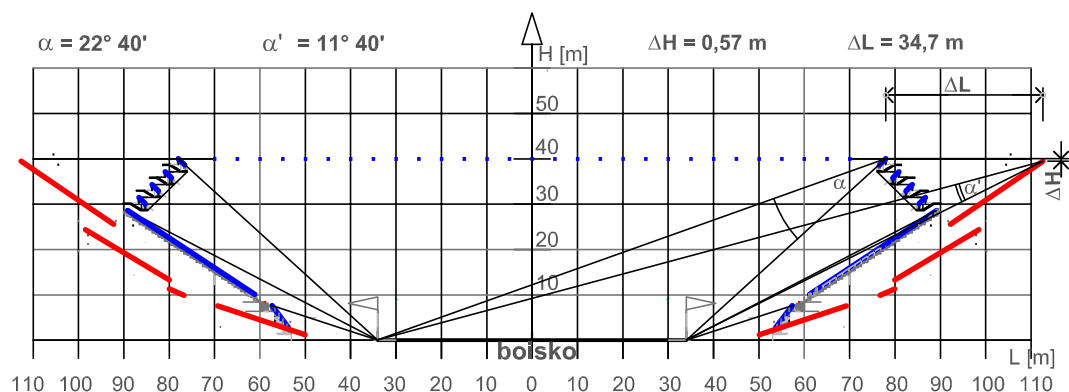
RYS. 5-25 ANALIZA PORÓWNAWCZA WŁAŚCIWOŚCI STROMEGO PROFILU MPS-1 I KLASYCZNEGO PROFILU STADIONU STADE DE FRANCE
