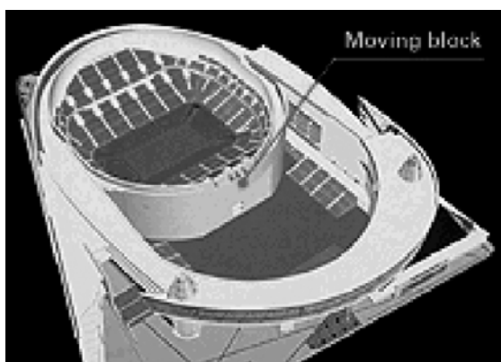
Fot. 1-15. Druga nagroda w konkursie architektonicznym na projekt Stadionu Narodowego Francji , Saint Denis, Paryż, architekt Jean Nouvel (1994). Koncepcja przekształcalnego stadionu z ruchomymi trybunami i ruchomym dachem areny, jako odpowiedź na wymogi piłkarskich i lekkoatletycznych funkcji stadionu.
