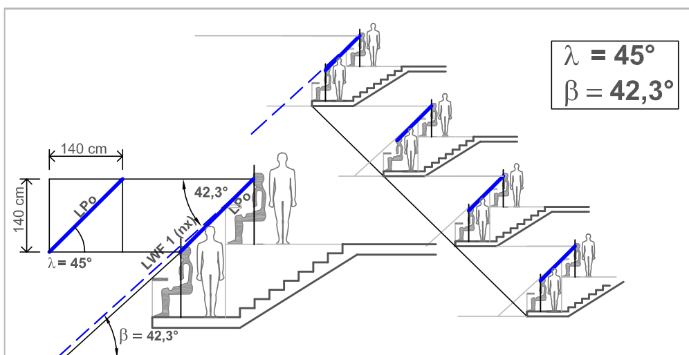
RYS. 5-23 MODUŁ FUNKCJONALNY MF 5 ( \lambda 45^\circ / \beta 42,3^\circ BALKON)
