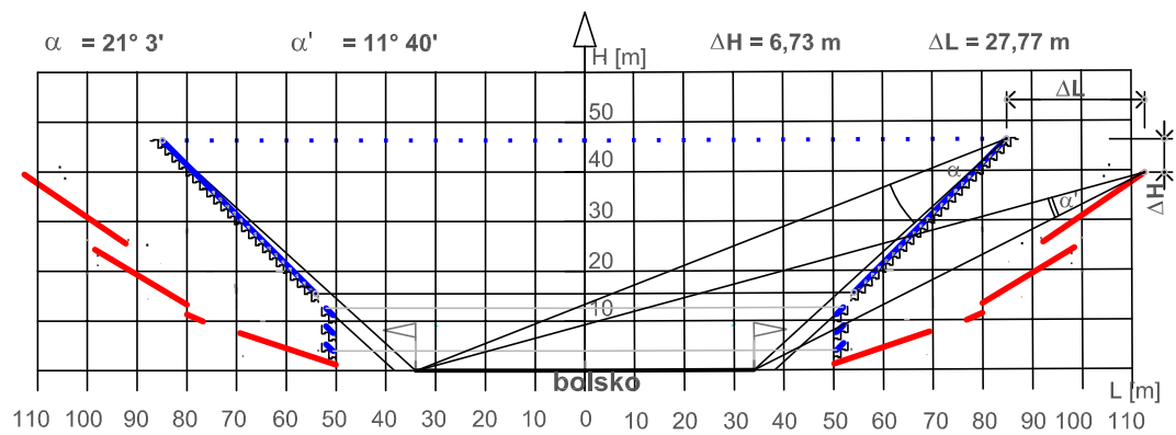
RYS. 5-29 ANALIZA PORÓWNAWCZA WŁAŚCIWOŚCI STROMEGO PROFILU MPS-3 I KLASYCZNEGO PROFILU STADIONU STADE DE FRANCE
