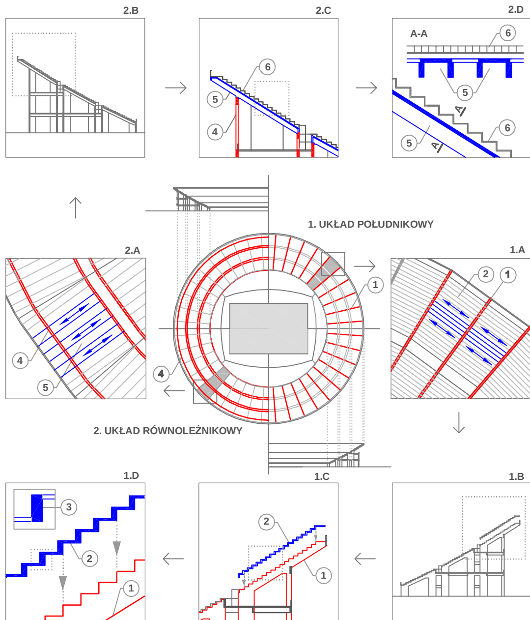
RYS. 5-7 UKŁAD KONSTRUKCJI WSPORCZEJ WIDOWNI: 1. Południkowy, 2. Równoleżnikowy
