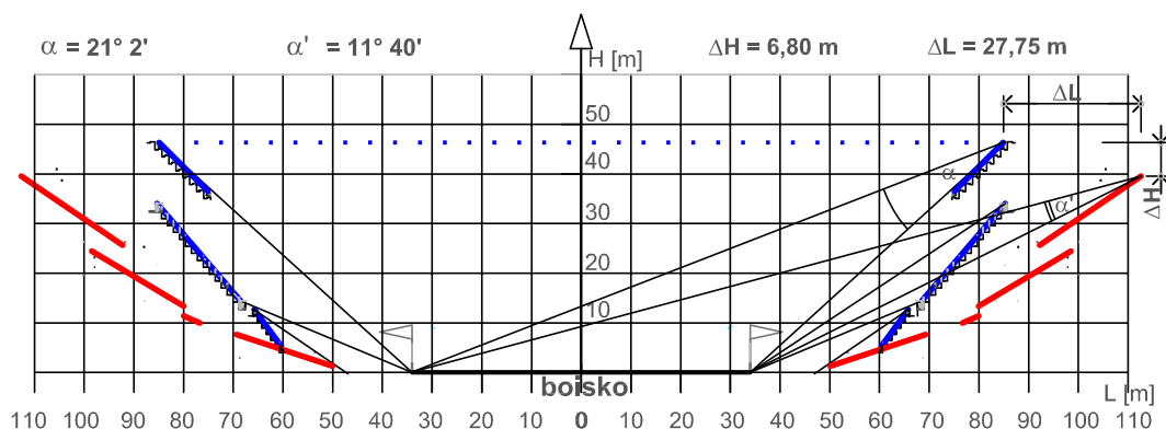
RYS. 5-27 ANALIZA PORÓWNAWCZA WŁAŚCIWOŚCI STROMEGO PROFILU MPS-2 I KLASYCZNEGO PROFILU STADIONU STADE DE FRANCE
