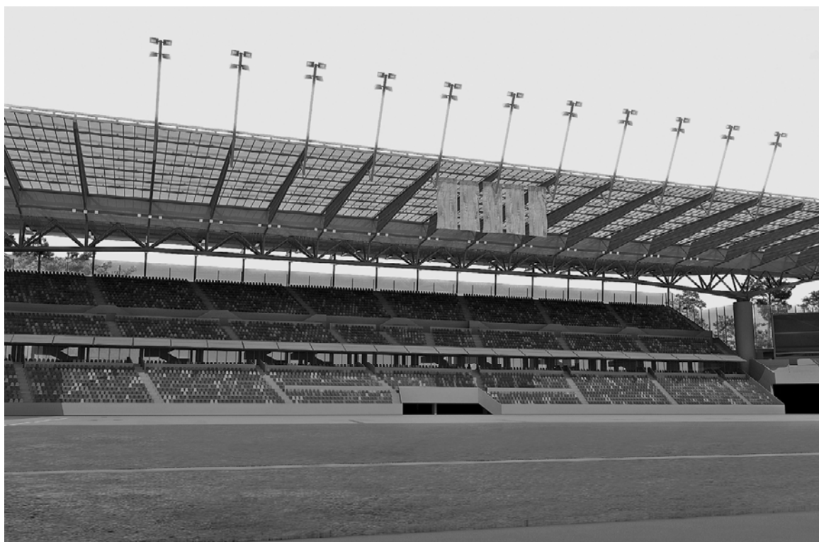
Fot. 5-3. Projekt koncepcyjny stadionu piłkarskiego Hetman w Białymstoku opracowany w ramach konkursu urbanistyczno-architektonicznego (Urząd Miejski w Białymstoku, 2007); autorzy: G. Dąbrowska-Milewska, J. Kabac, Z. Pelczarski, J. Żarnowiecka, M. Pelczarski (konstrukcja). W projekcie widowni zastosowano womitoria równoleżnikowe, ukośne układy schodów międzysektorowych i siedzisk oraz podłużny układ konstrukcji wsporczej. Wizualizacja: A. Babula, B. Dudziński.
