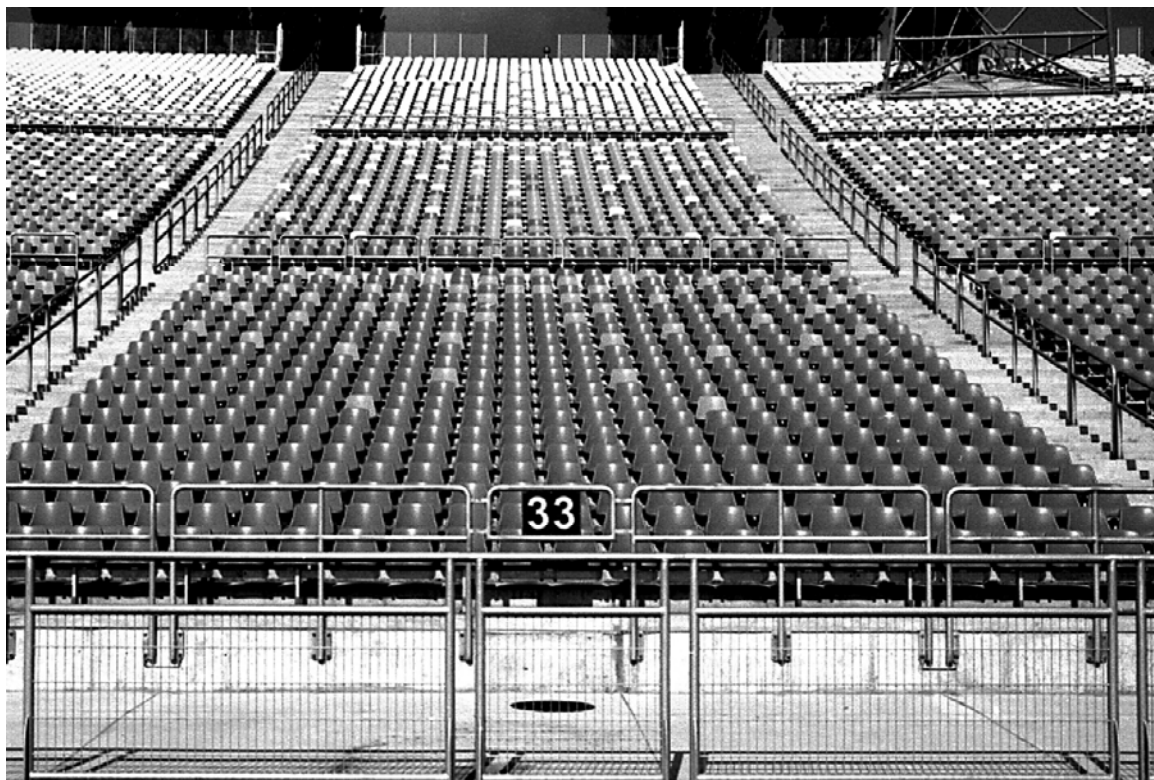
Fot. 2-11. Stadion Śląski, Chorzów, (1997). Widownia zachodnia. Przykład widowni łukowej o profilu krzywoliniowym. Widok z poziomu areny na sektor nr 33. Łukowa linia rzędów uzyskiwana jest w wyniku zastępowania teoretycznego łuku odcinkami linii prostej, stanowiącej cięciwy tego łuku. Szerokość sektora tworzona jest z trzech takich odcinków - czwartym jest odcinek ustalający szerokość schodów południkowych. Foto: autor.
