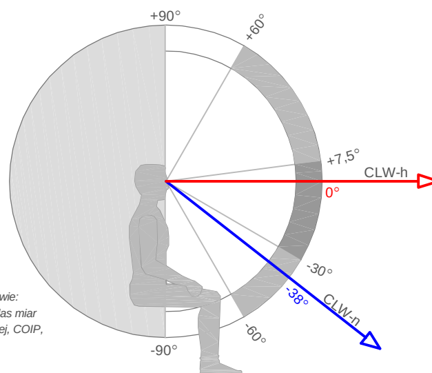
RYS. 1-9 PIONOWY ZAKRES WIDZENIA
