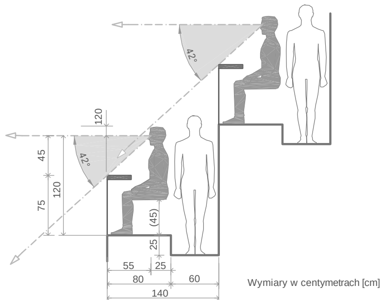
RYS. 5-2 TRYBUNA O PODWYŻSZONYM KOMFORTIE UŻYTKOWYM - RZĄD Z BLATEM CZOŁOWYM I OBNIŻONYM PRZEJŚCIEM Z TYŁU
