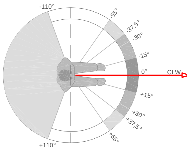
RYS. 1-8 POZIOMY ZAKRES WIDZENIA
