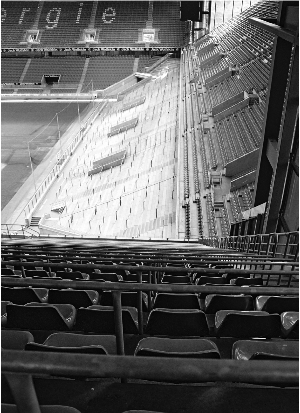
Fot. 2-7. RheinEnergie Stadion, Kolonia, (2004). Przykład widowni prostokątnej o profilu prostoliniowym. Nachylenie widowni górnej wynosi 35^\circ , co jest maksymalną normowo dopuszczalną wartością. Tak znaczna stromizna trybun wymagała zastosowania w każdym rzędzie balustrady czołowej. Niezwykłością prezentowanej widowni jest rozwiązanie trybun w rejonie narożnika boiska. Tak dalekie wysunięcie poza linię bramkową skrajnych miejsc powoduje, że mają one ekspozycję widokową nie na boisko lecz na prostopadłe trybuny. Nakierowanie centralnej linii widzenia na najbardziej skrajny narożnik obrazu pola boiska wymaga skrócenia tej osi o kąt dochodzący do wartości ok. 67^\circ . Foto: autor.
