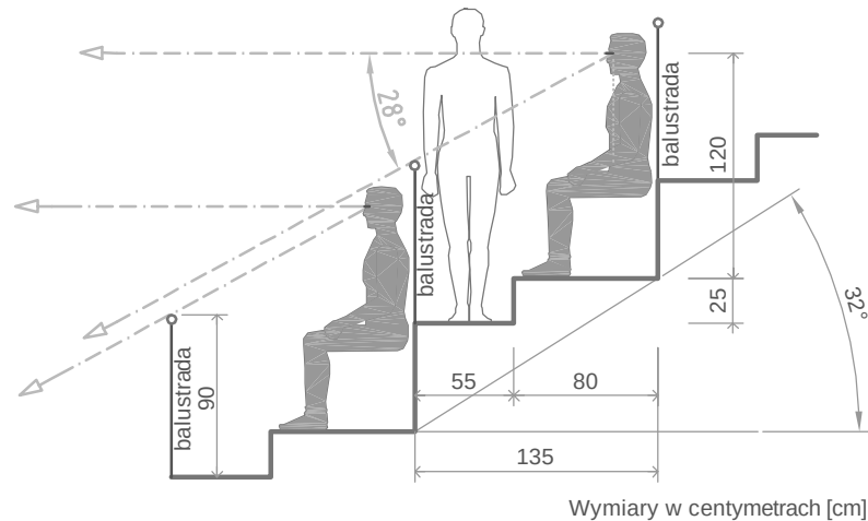
RYS. 5-1 TRYBUNA O PODWYŻSZONYM KOMFORTIE UŻYTKOWYM - RZĄD Z BALUSTRADĄ I OBNIŻONYM PRZEJŚCIEM Z PRZODU
