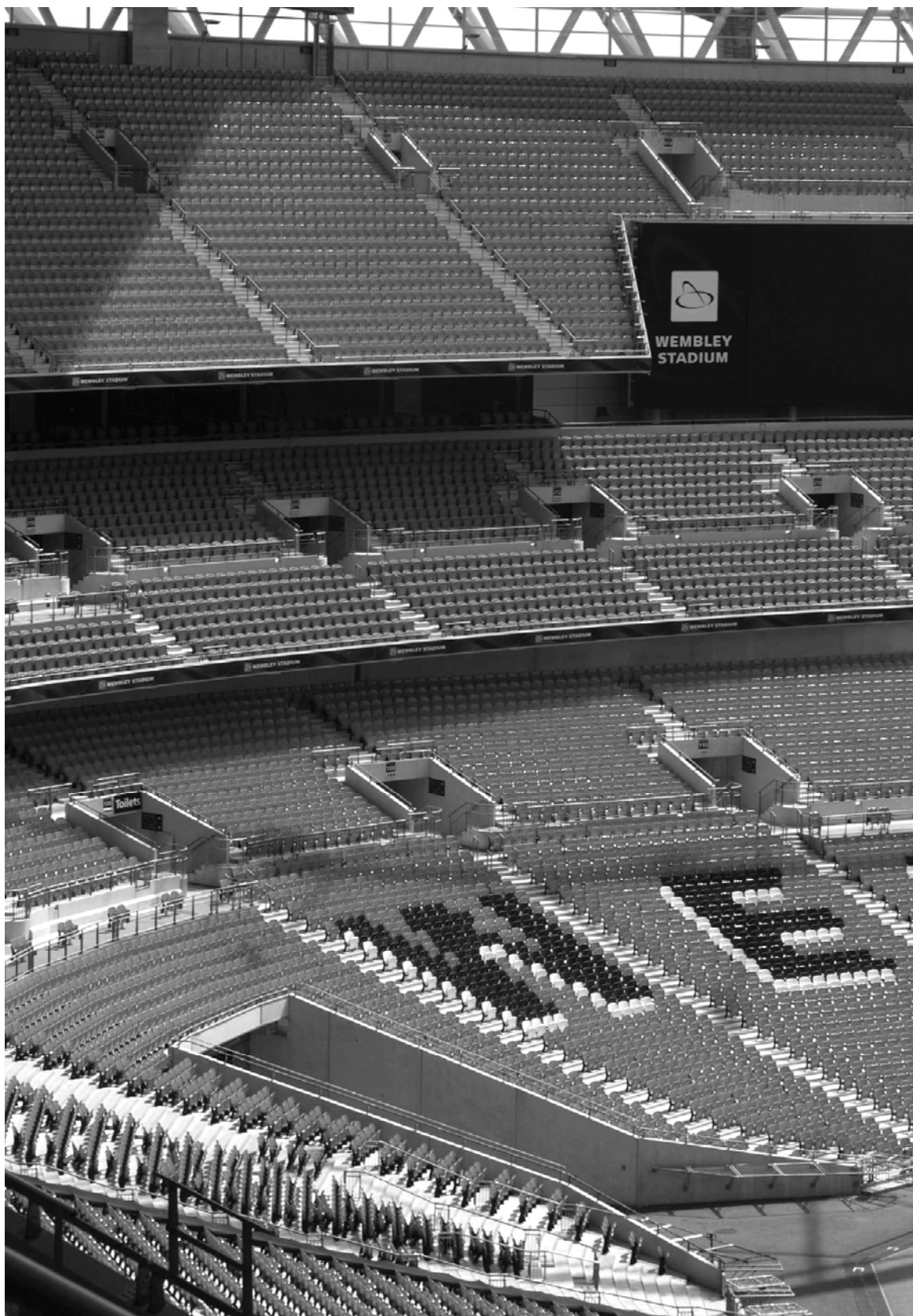
Fot. 2-8. New Wembley Stadium , Londyn, (2007). Trzypiętrowa widownia o profilu prostoliniowym o zróżnicowanym układzie rzędów w rzucie poziomym. Widownia dolna posiada cechy typowej widowni prostokątnej, piętro drugie i trzecie charakteryzuje układ prostokątny wzdłuż boków boiska i układ łukowy w strefach zabramkowych. Dolne piętra mają dobrze rozwinięty system komunikacyjno-ewakuacyjny, podczas gdy piętro najwyższe cechują w tym względzie znacznie gorsze parametry. Przykład interesującego rozwiązania womitoriów, zapewniającego dobrą segregację ruchu. Foto: M. Pelczarski.
