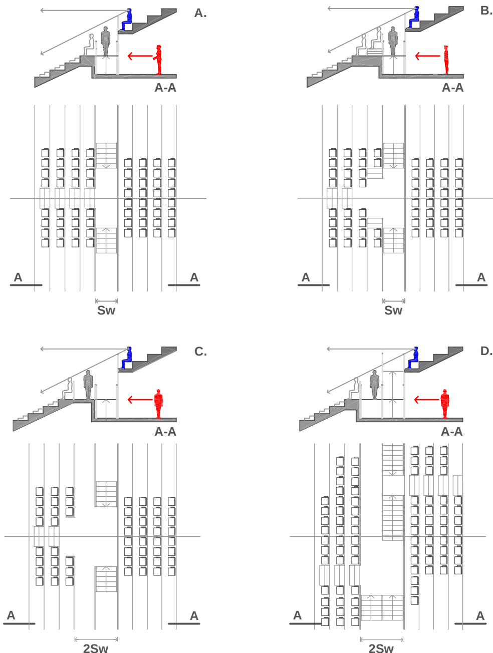
RYS. 5-6 WOMITORIA RÓWNOLEŻNIKOWE
