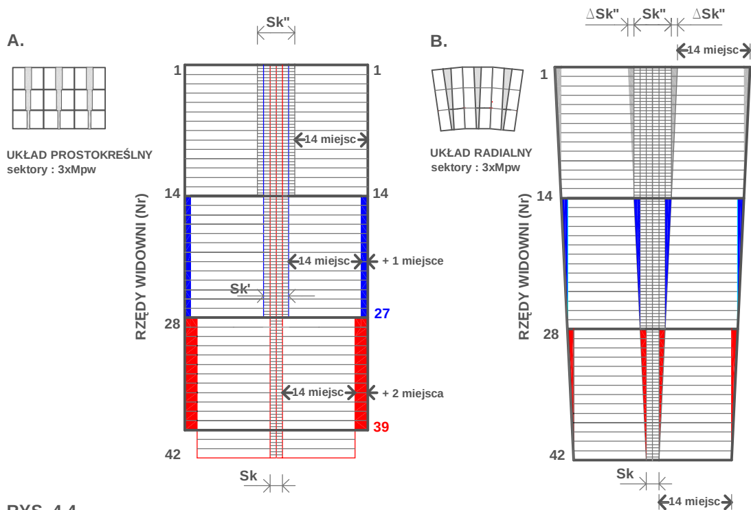
RYS. 4-4 ◀14 miejsc▶ PRZYKŁAD KSZTAŁTOWANIA POWTARZALNEGO SEKTORA WIDOWNI Z ZASTOSOWANIEM EWAKUACYJNEGO MODUŁU POJEMNOŚCI. A. Transformacja sektora 3xMpw dla widowni o układzie prostokreślnym. B. Transformacja sektora 3xMpw dla widowni o układzie radialnym
