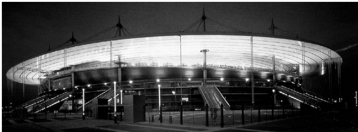
Fot. 1-14. Stade de France , Paryż (1998). Realizacja pierwszej nagrody w konkursie architektonicznym na Narodowy Stadion Francji . Unikalna forma i konstrukcja dachu zawieszonego na dwudziestu słupach nośnych – równoważona zewnętrznymi odciegami kablowymi. Foto: reprodukcja z broszury promocyjnej Komitetu Organizacyjnego MŚ – FIFA, Francja 1998.
