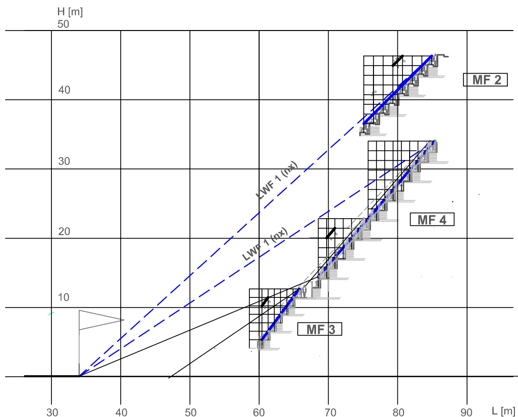
RYS. 5-26 MODEL PROFILU STROMEGO MPS 2 (Złożenie modułów MF 3, MF 4 i MF 2)
