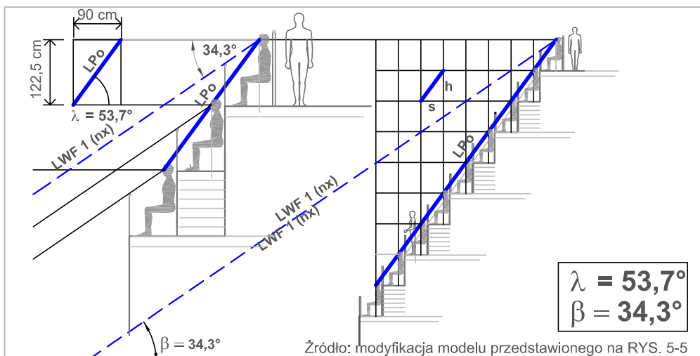
RYS. 5-21 MODUŁ FUNKCJONALNY MF 3 ( \lambda 53,7^\circ / \beta 34,3^\circ )
