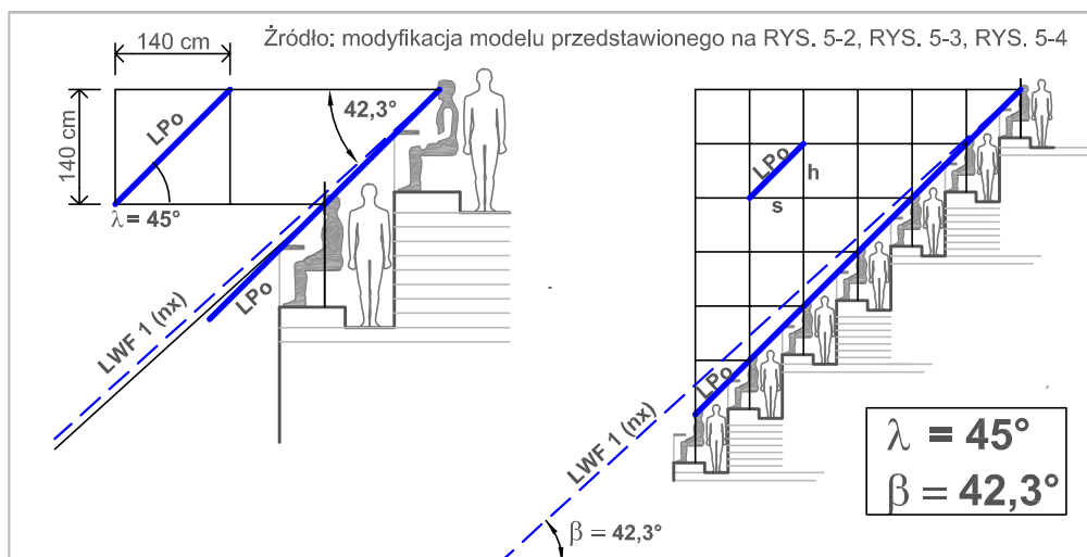
RYS. 5-20 MODUŁ FUNKCJONALNY MF 2 ( \lambda 45^\circ/\beta 42,3^\circ )
