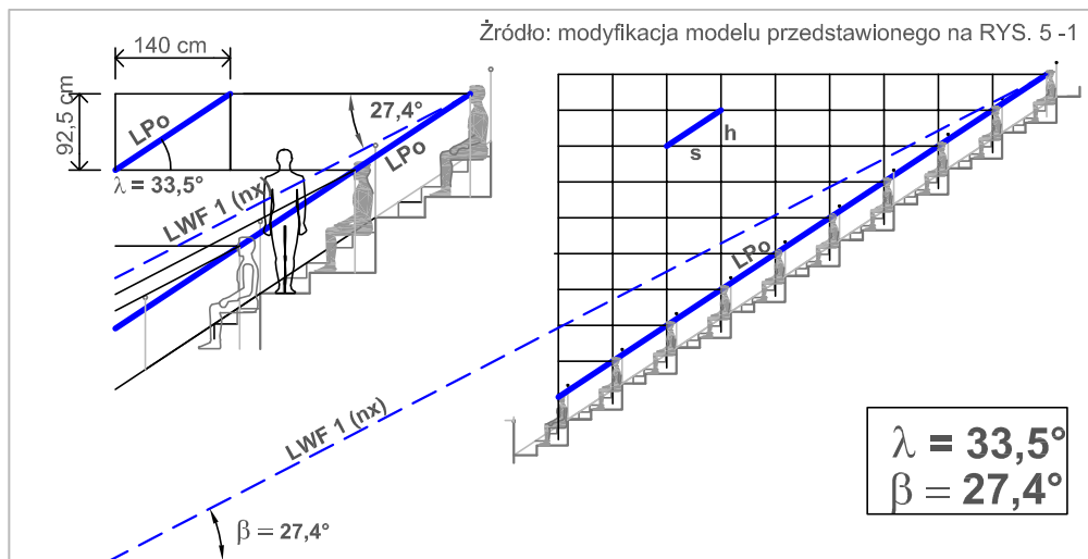
RYS. 5-19 MODUŁ FUNKCJONALNY MF 1 ( \lambda 33,5^\circ/\beta 27,4^\circ )
