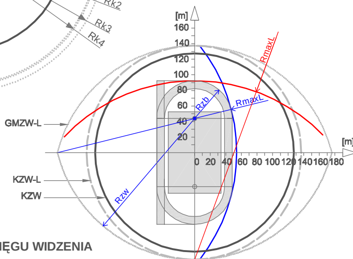
RYS. 1-13 KOŁA MAKSYMALNYCH ZASIĘGÓW WIDZENIA DLA GIER WIELKIEGO POLA I DUŻEJ PIŁKI
