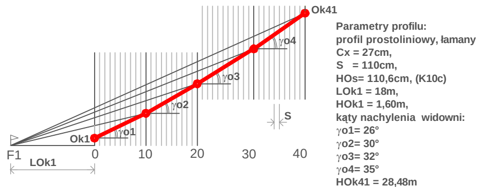
RYS. 2-40 PRZYKŁADOWY PROFIL WIDOWNI SPEŁNIAJĄCEJ WARUNEK NIEZAKŁÓCONEJ WIDOCZNOŚCI LINII FOKUSÓW BLIŻSZYCH DLA CAŁEGO SPEKTRUM K10c-M95c ANTROPOMETRYCZNEJ WYSOKOŚCI OCZNEJ POPULACJI POLSKIEJ
