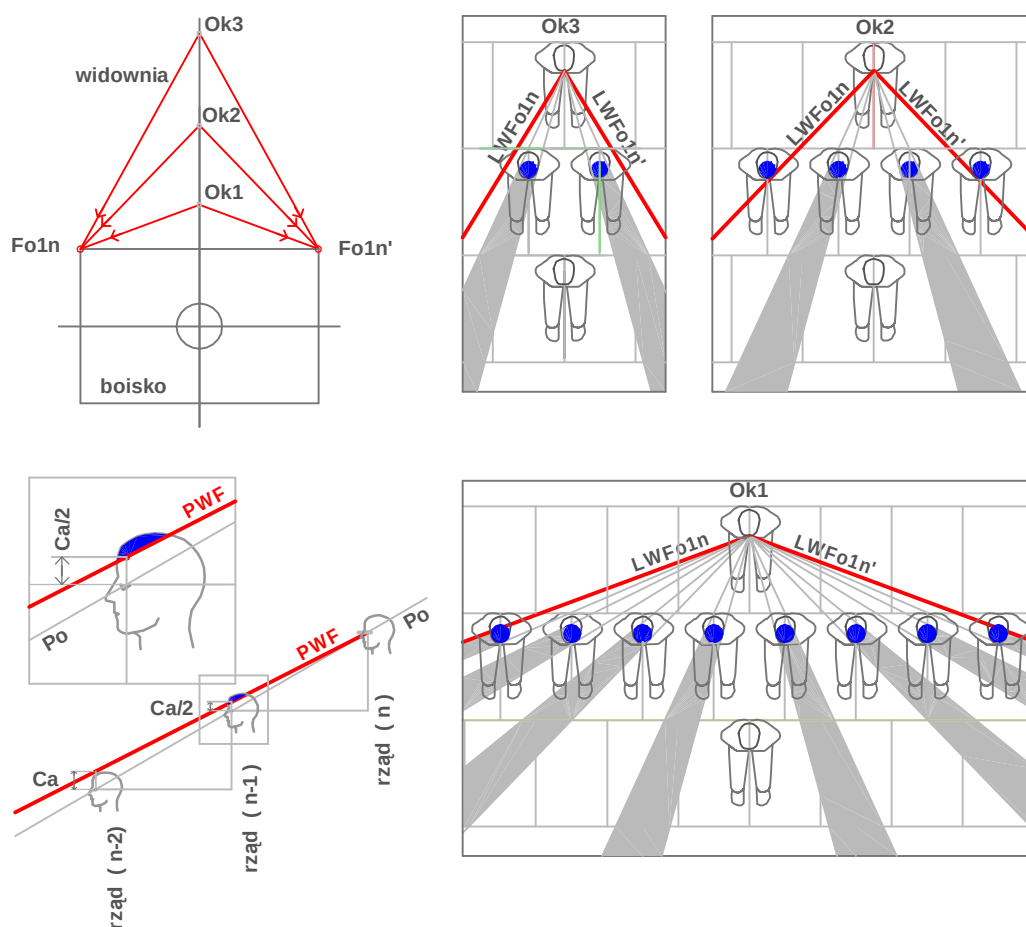
RYS. 2-32 PROFIL WIDOWNI O NAPRZEMIENNYM (SZACHOWNICOWYM) UKŁADZIE SIEDZISK I PRZEWYŻSZENIU NOMINALNYM Ca=12\text{cm} CO DRUGI RZĄD. ANALIZA WIDOCZNOŚCI LINII FOKUSÓW BLIŻSZYCH
