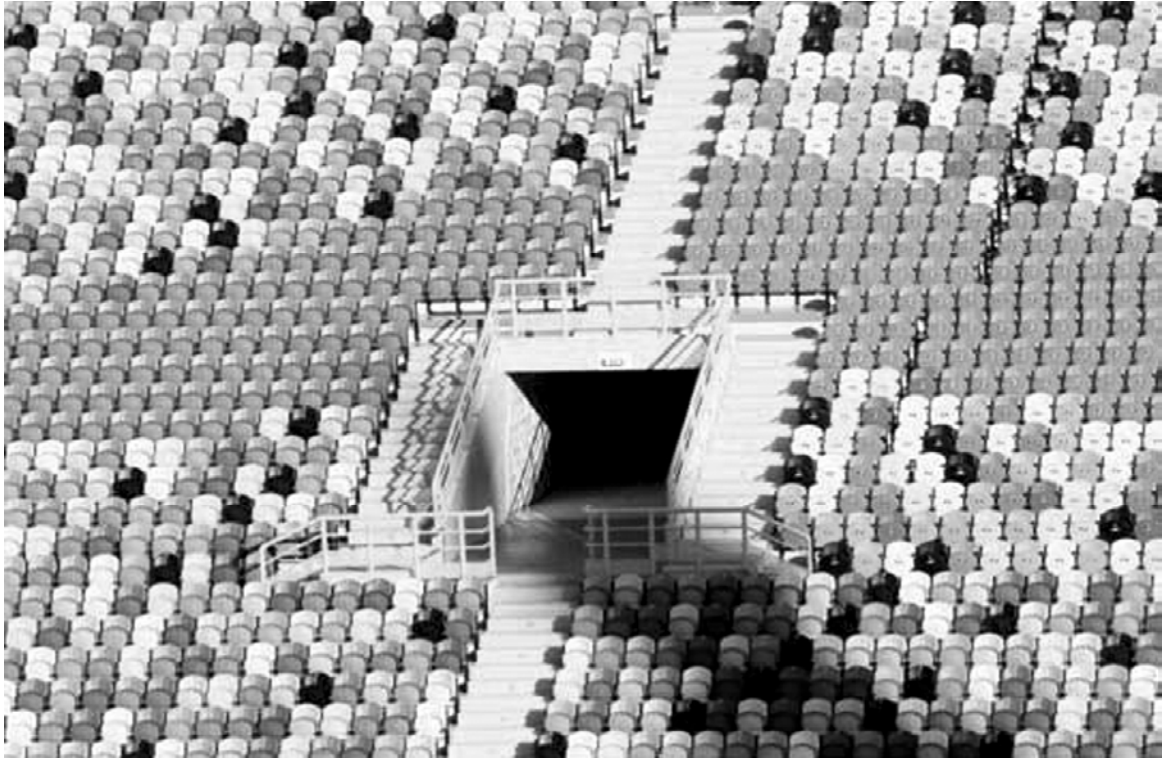
Fot. 4-6. Stadion im. Jose Alvalade, Lisboa. Fragment widowni – przykład aranżacji z osiowym układem schodów południkowych nad i poniżej womitorium. System pozwala na segregację pasm ruchu widzów w obrębie przestrzeni womitorium.
