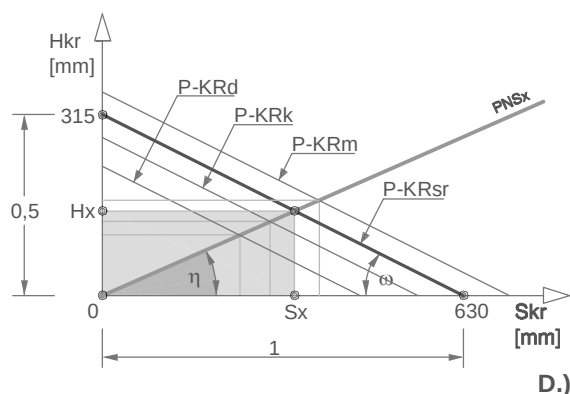
RYS. 3-1 TEORETYCZNE PODSTAWY GEOMETRII SCHODÓW WYGODNYCH. RÓWNANIE BLONDELA : "2H + S = DŁUGOŚĆ KROKU"
