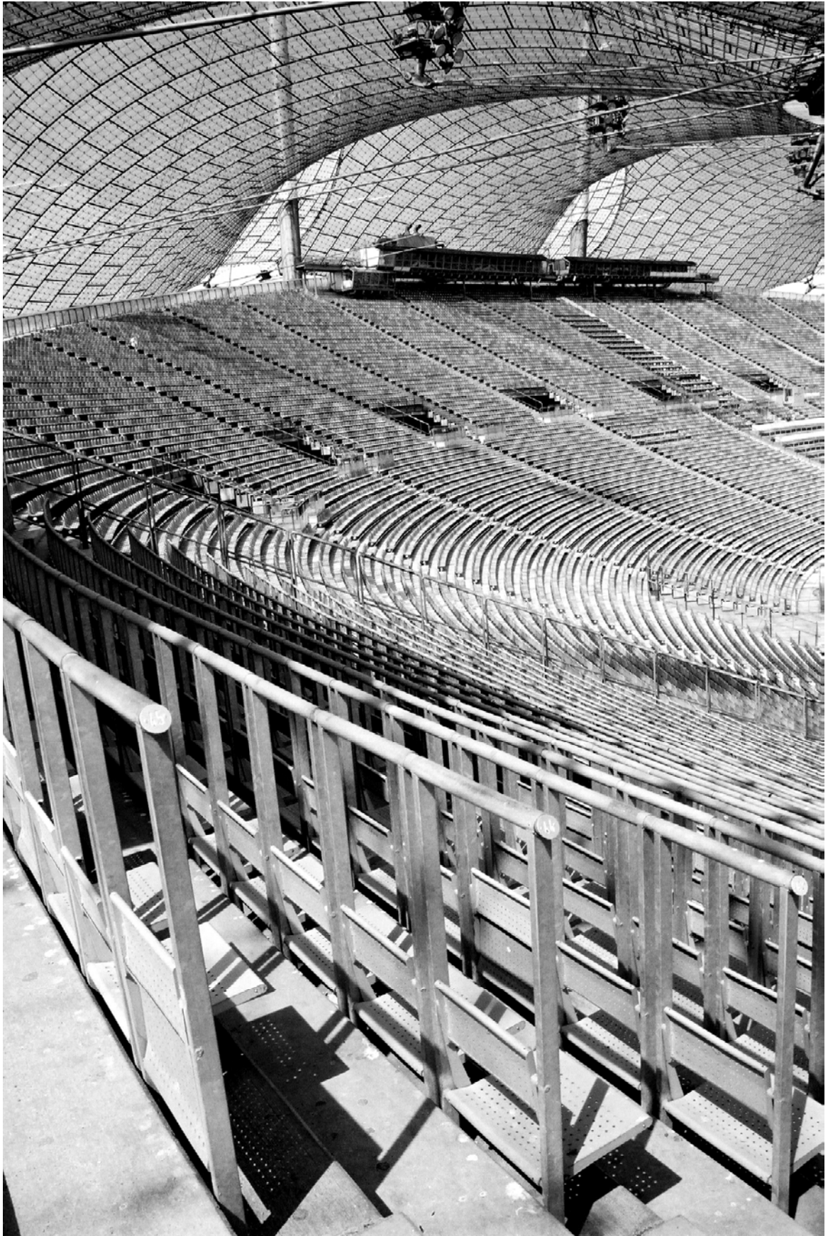
Fot. 5-1. Stadion Olimpijski w Monachium – stan w roku 2006. Na pierwszym planie sektor widowni za bramkowej, jako przykład sposobu kształtowania miejsc umożliwiających zamiennie przyjmowanie pozycji stojącej lub siedzącej.
