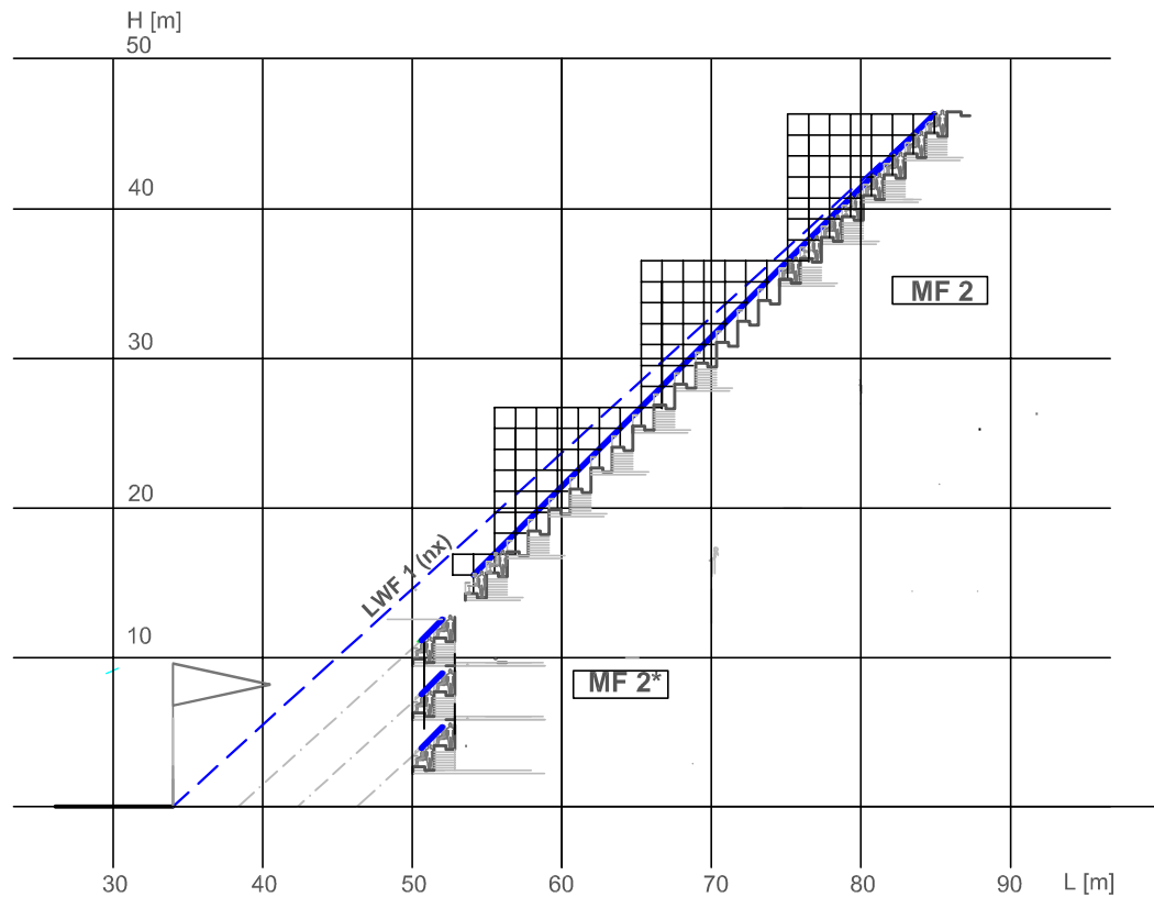
RYS. 5-28 MODEL PROFILU STROMEGO MPS 3 (Złożenie modułów MF 2* i MF 2)
