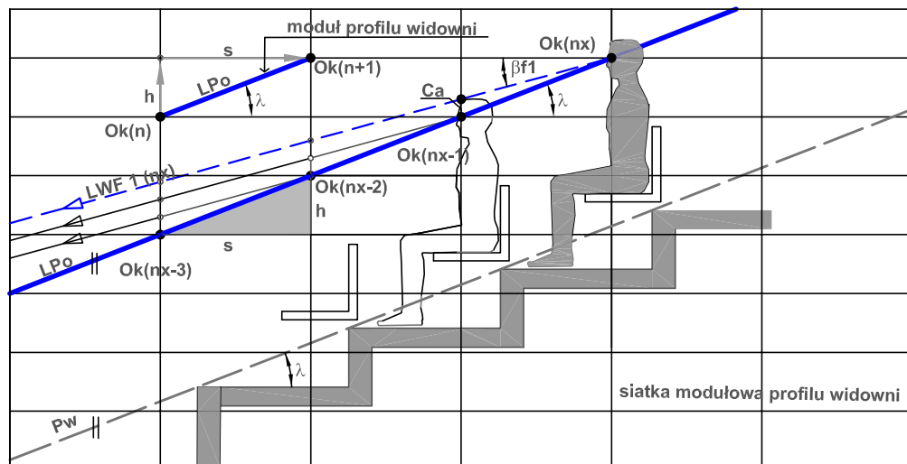
RYŚ. 5-17 LINIA PŁASZCZYZNY OCZNEJ JAKO LINIA PROFILU WIDOWNI. DEFINICJA MODUŁU PROFILU WIDOWNI
