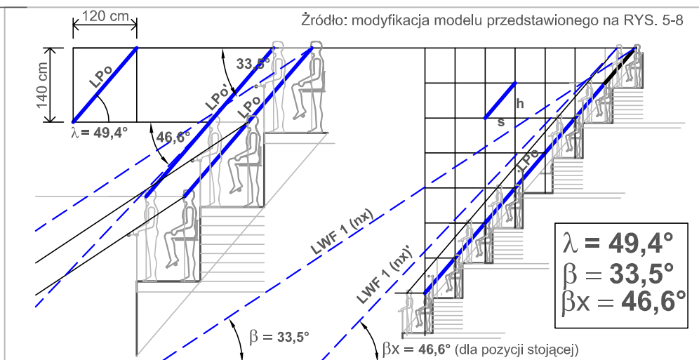
RYS. 5-22 MODUŁ FUNKCJONALNY MF 4 ( \lambda 49,4^\circ / \beta 33,5^\circ / \beta x 46,6^\circ )
