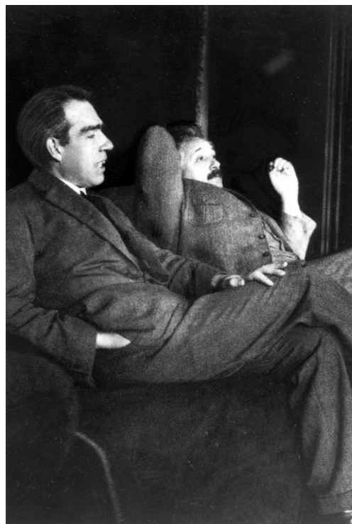
Niels Bohra i Albert Einstein w domu Paula Ehrenfesta w Leiden (grudzień 1925)
