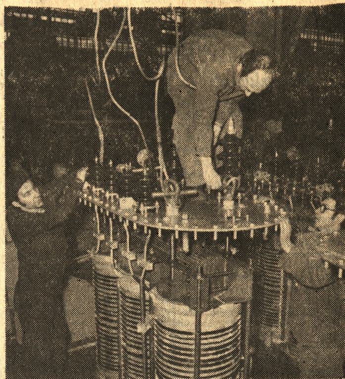
Pierwszy transformator wyprodukowany na licencji austriackiej firmy „Elin”, opuścił tódką Fabrykę Transformatorów i Aparatury Trakcyjnej „Elta” przed szesnastu laty. W oparciu o tę licencję opracowano i wykonano całą rodzinę transformatorów własnej konstrukcji. Pracują one we wszystkich elektrowniach budowanych po 1965 roku — m. in. w Turoszowie, Patnowie, Rybniku, Koźlenicach. Od kilku lat transformatory z „Elty” trafiają także na eksport — m. in. do Japońsk, Iraku, Turcji, Algierii. W tym roku zakład wyprodukuje łącznie około 10 000 sztuk urządzeń. CAF — fot. A. Zbraniecki
