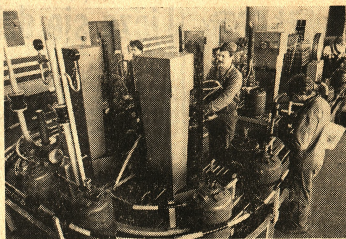
Wojewódzkie Przedsiębiorstwo Gospodarki Komunalnej i Mieszkaniowej w Koninie uruchomiło rozlewnię gazu. Zakład, wyposażony w nowoczesne duńskie urządzenia do napełniania butli, dostarcza gaz do gospodarstw i przemysłu całego województwa. Fot. — R. Królak
