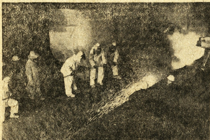
W Katowickim pracuje jeden z najnowocześniejszych obiektów metalurgicznych na świecie — Huta „Katowice”. Obecnie trwa jej drugi etap budowy. Na zdjęciu: historyczny już moment — pierwszy spust surowki. CAF — fot. Jakubowski
