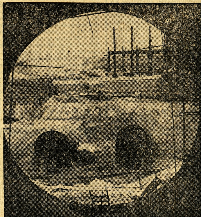
Nad jeziorem Żarnowieckim w Gdańsku powstaje kolejna elektrownia szczytowo-pompowa. Pierwszy turbozespół o mocy 1700 MW w elektrowni „Żarnowiec” zasili krajowy system energetyczny w roku 1980.
