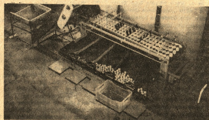
Na zdjęciu: Sortownik diafragmowy do pomidorów o wydajności 5 ton na godzinę. Fot. Archiwum
