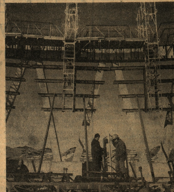
Wraz z budową kopalni w Bełchatowie trwa wznoszenie elektrowni. Obecnie prowadzone są prace przy montażu konstrukcji stalowej wieży nośnej koła nr 1. Kontynuowana jest budowa chłodni. Na zdjęciu: podczas montażu konstrukcji chłodni. CAF — fot. Zbraniecki
