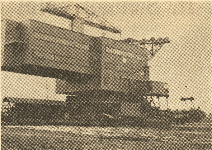
Koparka, która była nieprzydatna w Turowie, została przez brygadę KZN wyremontowana i pracuje już we Władysławowie. Fot. — Archiwum
