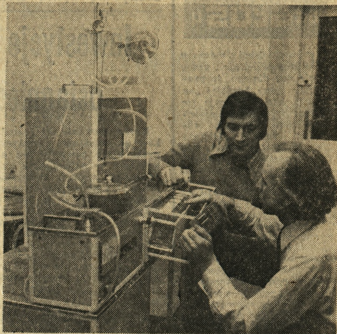
W Zakładach Elektronicznej Aparatury Medycznej w Zabrzu rozpoczęto seryjną produkcję aparatu zwanego „szluzową nerką”. Pierwszą serię 25 aparatów otrzymała krajowa służba zdrowia. Na zdjęciu — podczas prób urządzenia. CAF — fot. Jakubowski
