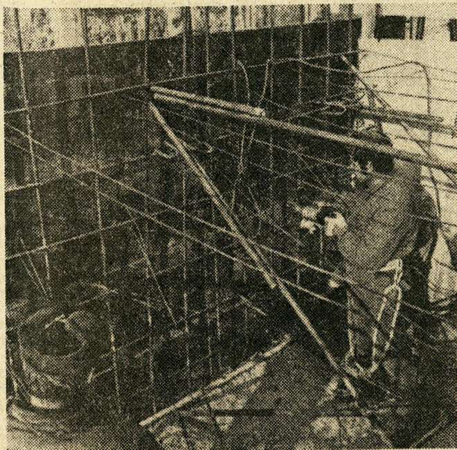
Brygady „Energopolu II”, pracujące przy budowie zbiornika wodnego na Dunajcu koło Niedzicy, prowadzą roboty żelbetowe, cięśliarskie i ziemne. Inwestycja ta zaliczana jest do szczególnie ważnych w gospodarce narodowej i stanowi jeden z etapów regulacji gospodarki wodnej w kraju.
