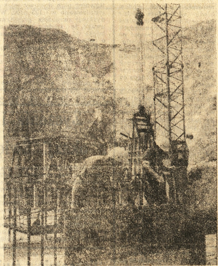
Na Dunajcu koło Czorsztyna powstaje zbiornik wodny o pojemności 250 milionów metrów sześciennych. Zbiornik ten obok zadań przeciwpowodziowych, w razie potrzeby będzie zasilał w wodę elektrownię Póleniec. Na zdjęciu: budowa wlotów do sztolni energetycznych. CAF — fot. Monot
