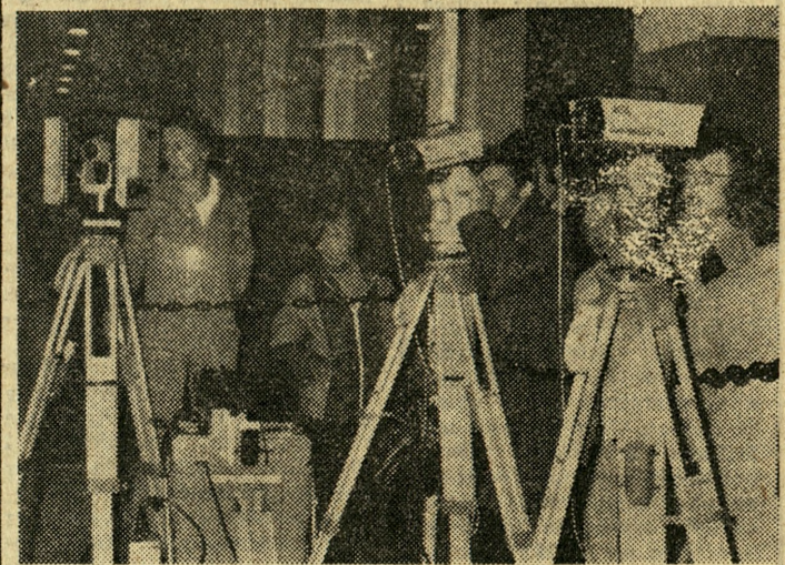
Szwecja prezentuje m. in. niezwykle precyzyjne urządzenia przydatne szczególnie w geodezji, kartografii i fotogrametrii. Działają one na zasadzie wiązki laserowej lub promieni podczerwonych.
