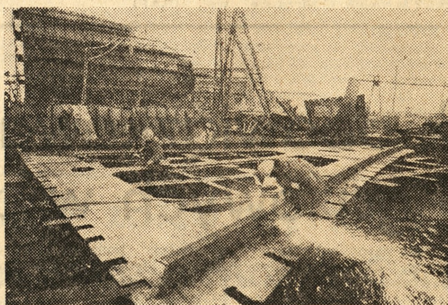
Na zdjęciu: prace przy budowie kolejnych sekcji m/s „Walka Młodych”.
