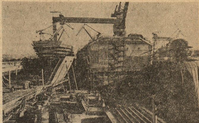
W drugim suchym doku Stoczni im. Komuny Paryskiej w Gdyni trwa budowa pierwszego statku. Jest to gazowiec typu LPG, przeznaczony dla armatora zagranicznego. Na zdjęciu: prace przy montażu gazowca. Fot. — CAF
