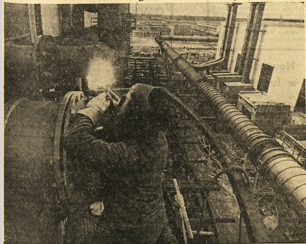
Pod Głogowem dobiega końca budowa drugiej huty miedzi. Trwają ostatnie prace montażowe w hłenowni oraz w części zwanej ogniwą. Roboty wykonują specjaliści wielu krajowych przedsiębiorstw. Na zdjęciu: spawacz Kazimierz Maciejewski z poznańskiego „Mostostalu” montuje instalację rurową hłenowni.
