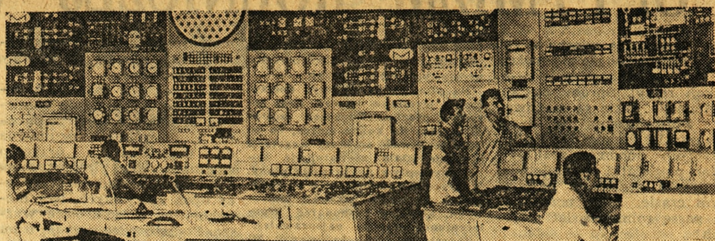
Nowoworonecka Elektrownia Atomowa w ZSRR jest jedną z największych na świecie. Jest ona ośrodkiem naukowym energetyki jądrowej, w którym podnoszą kwalifikacje nie tylko specjaliści ze Związku Radzieckiego, lecz także z krajów RWPG. Na zdjęciu: pulpity sterownicze bloku energetycznego w elektrowni atomowej. Fot. — CAF
