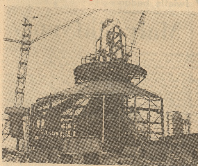
Tak wygląda konstrukcja przyszłego wielkiego pieca. Trzeba widać autorowi tego zdjęcia, że na dachu są ludzie — monterzy. Ale to tak daleko, tak wysoko, że na fotografii nie sposób ich zauważyć.
