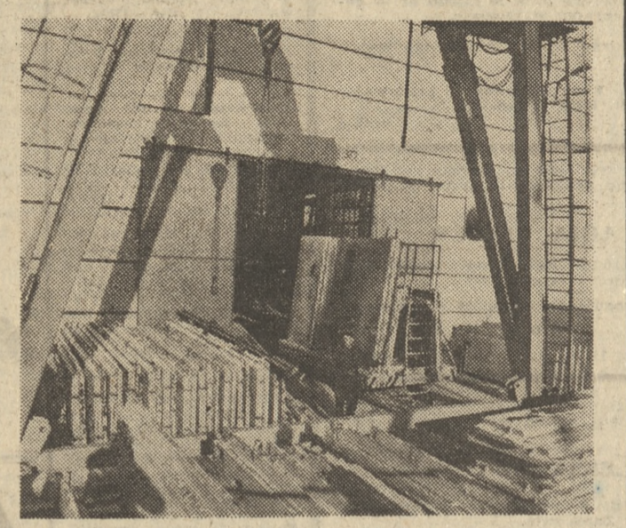
Nowo zbudowana w Obornikach „fabryka domów” (Zakład Prefabrykacji Betonowej) przygotowuje różne elementy dla budownictwa wiejskiego. Zbudowana w 11 miesięcy, wytwarza teraz rocznie około 13 000 m sześć. ścian i stropów, wystarczających na zmontowanie 3 250 izb mieszkalnych. CAF — fot. Staszyszyn
