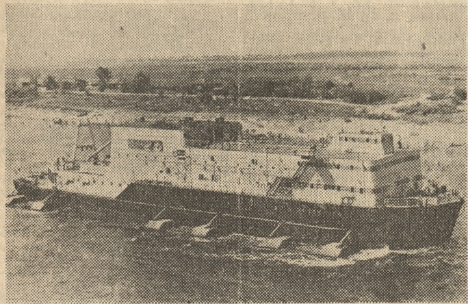
Pływające elektrownie „Zorza Polarna”, są niezastąpione na Dalekiej Północy, w pobliżu nowoodkrytych złóż surowcowych. Siłak — elektrownia ma specjalną instalację, która zapobiega wmarzaniu kadiuba w lód.
