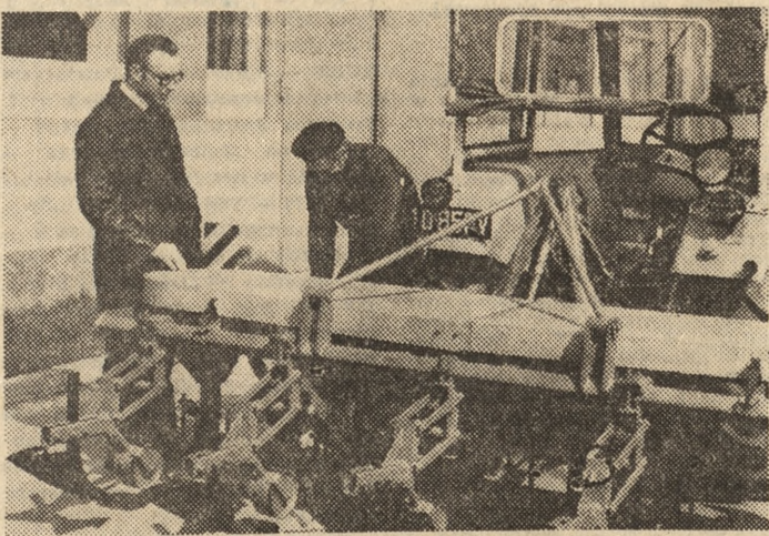
Obsypnik do ziemniaków sprzężony z aktywnym spulchniaczem gleby. Patent Politechniki Poznańskiej. Urządzenie zostało zaprojektowane przez doc. dra Kazimierza Mielca i doc. dra Zdzisława Kośmickiego. Na zdjęciu: dyrektor PIMR doc. dr K. Mielec oraz mechanik Henryk Zgola.
