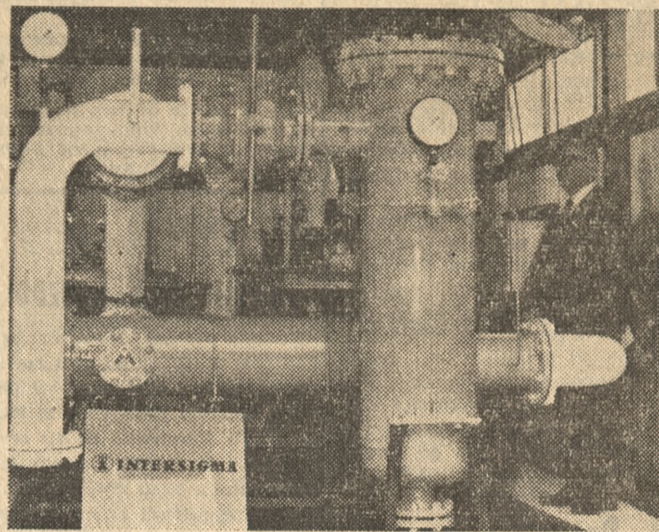
Stacja redukcyjno-pomiarowa dla gazu ziemnego demonstrowana w pawilonie Czechosłowacji jest jednym z większych eksponatów. Dotychczas handlowcy polscy zakupili 5 takich urządzeń.
