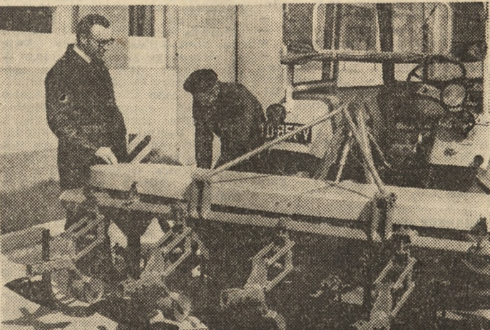
Obsypnik do ziemniaków sprzężony z aktywnym spulchniaczem gleby. Patent Politechniki Poznańskiej. Urządzenie zostało zaprojektowane przez doc. dra Kazimierza Mielca i doc. dra Zdzisława Kośmickiego. Na zdjęciu: dyrektor PIMR doc. dr K. Mielec oraz mechanik Henryk Zgola.
