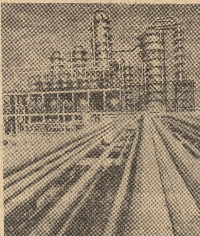
Nowa rafineria w Szazhalombatta, uruchomiona w listopadzie ubr. osiągnie roczną wydajność 3 milionów ton. Fot. — CAF
