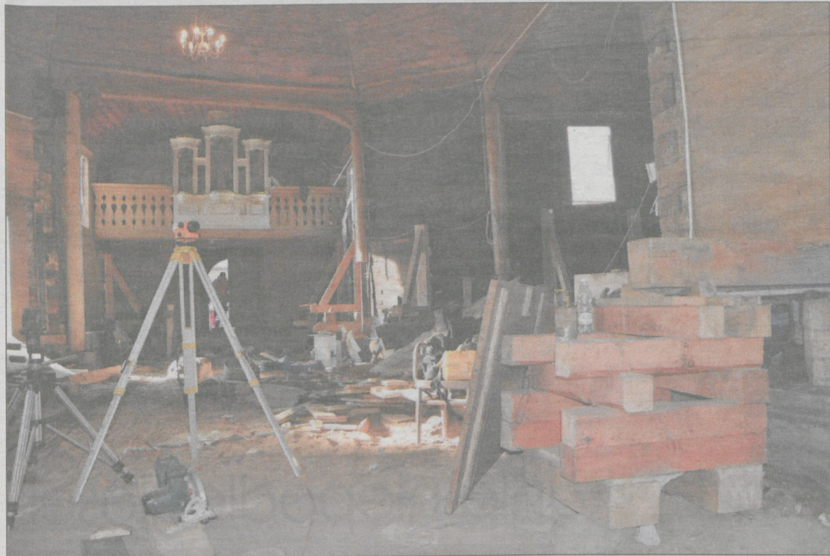
Z wnętrza wybrano metr piasku. Ścianę najpierw oparto na przyporze i stosie belek. Później (z prawej) montuje się podnośniki kozłowe, które zastąpią przyporę. Na końcu umieszczona zostanie podwalina
