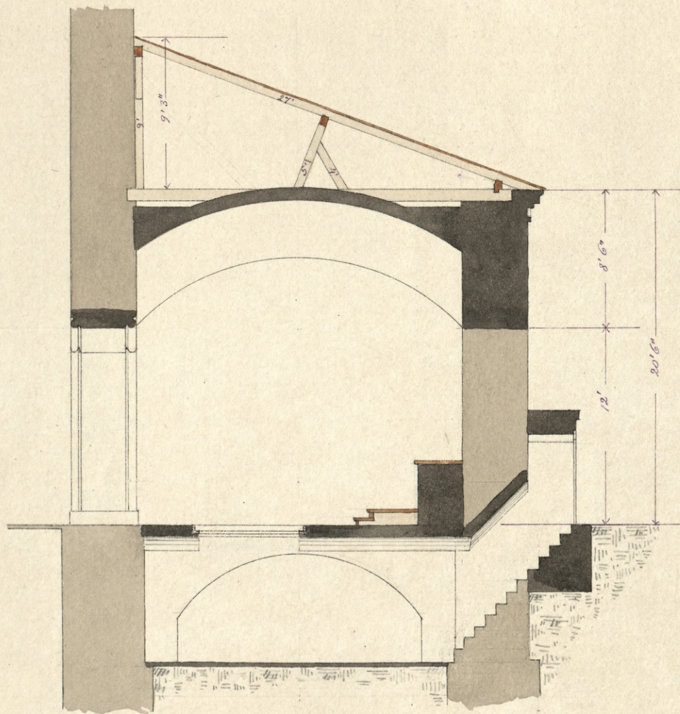
Przekrój AB
