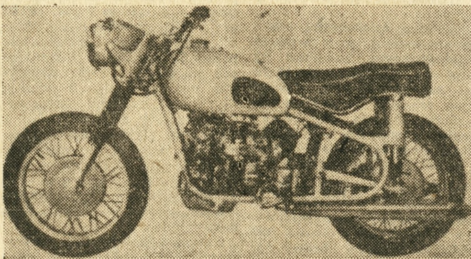
Motocykl BMW z silnikiem NSU-Wankel Spider o mocy 50 KM z pojemnością 2x500 ccm. Silnik zamocowany jest w podwójnej ramie. Na zdjęciu motocykl nie ma chłodnicy.
