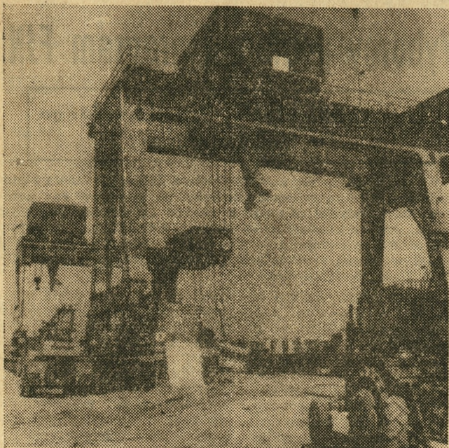
22 lipca br. ruszą we Włocławku agregaty największej w kraju nizinnej zapory i siłowni wodnej, stanowiących główne ogniwo systemu stopni wodnych kaskady do dolnej Wisły. Na „Dzień Budowlanych” zostanie oddana do użytku kolejna część zapory — śluza wraz z awanportem. — Oto potężne dzwigi bramowe służące do montażu śluz i agregatów hydroelektrowni. CAF — Gill — Telefoto
