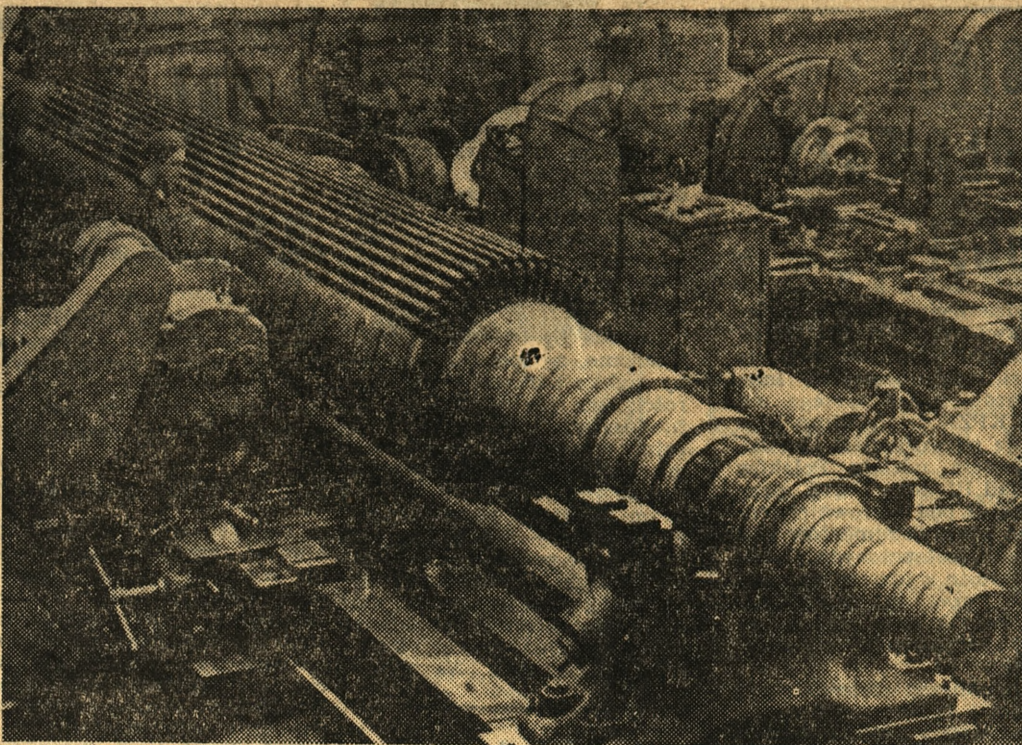
Na zdjęciu: rotor turbogenerators o mocy 500.000 kW produkowany w leningradzkiej fabryce „Elektrosila”.
