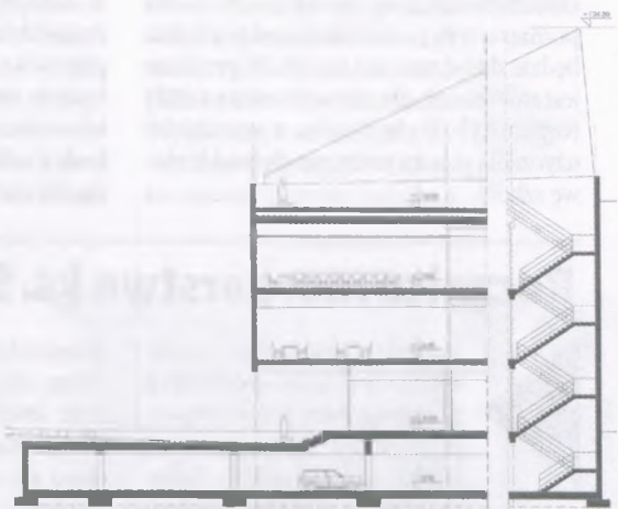
Przekrój poprzeczny budynku z podziemnym parkingiem oprac. Magdalena Malepszak
