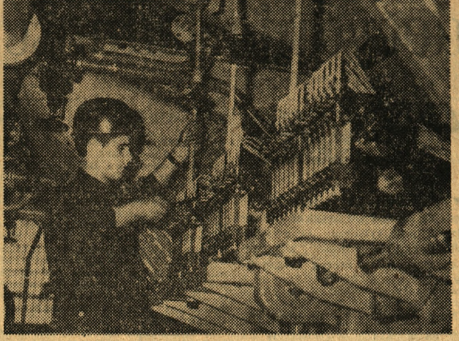
Po zakończeniu produkcji parowozów w 1958 r. rozpoczęto budowę silników okrętowych, opartą na licencjach szwajcarskiej, duńskiej i polskiej. Oprócz silników okrętowych dostarczanych na statki budowane w stocznich polskich, kilka z nich przeznaczono na eksport bezpośredni do NRD i Jugosławii. Na zdjęciu — montaż przewodów smarowania cylindrów silnika okrętowego.
