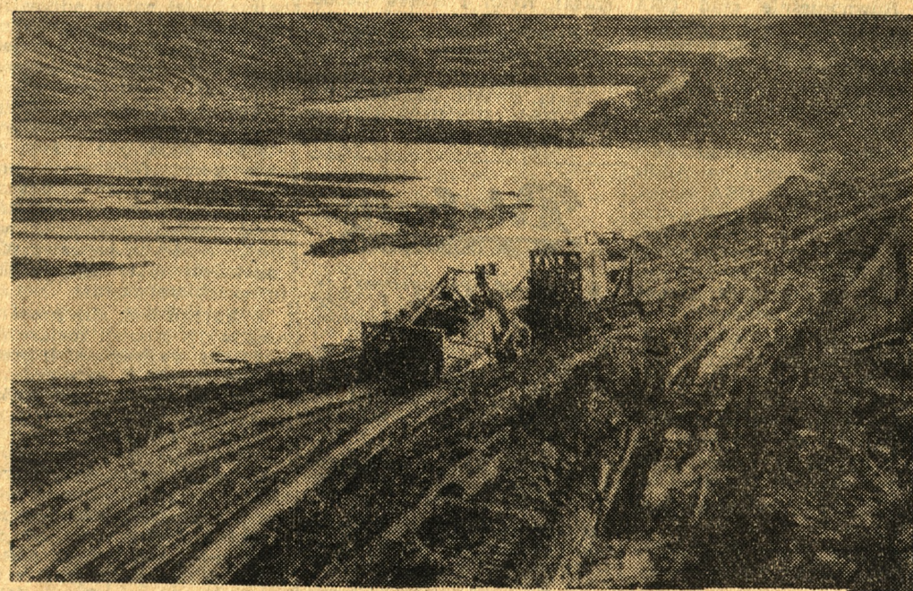
Prace przy nowym korycie. Warty w Poznaniu
