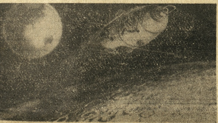
Wykonany przez grafika agencji TASS rysunek przedstawia radziecką stację kosmiczną „LUNA-10“ na orbicie okołosieciowej.
