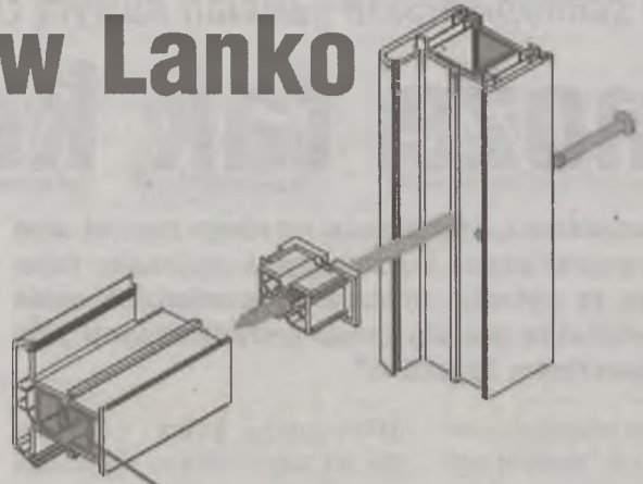
Wzmocnienie stalowe NA 44 zwiększające sztywność całego okna poprzez połączenie z ramą system ten jest opatentowanym rozwiązaniem przez firmę DECEUNINCK wykorzystywanym przez producenta okien i drzwi LANKO
