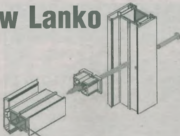
Wzmocnienie stalowe NA 44 zwiężkające sztywność całego okna poprzez połączenie z ramą system ten jest opatentowanym rozwiązaniem przez firmę DECEUNICK wykorzystywanym przez producenta okien i drzwi LANKO.
