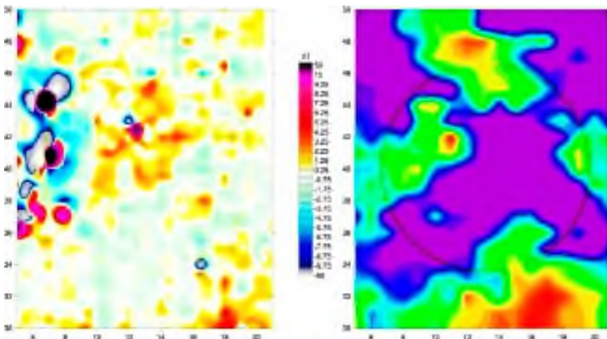
Ryc. 11. Rejon 1. Porównanie map ilustrujących rezultaty prospekcji gradiometrycznej metodą magnetyczną (lewa) i elektroporowej (prawa)
