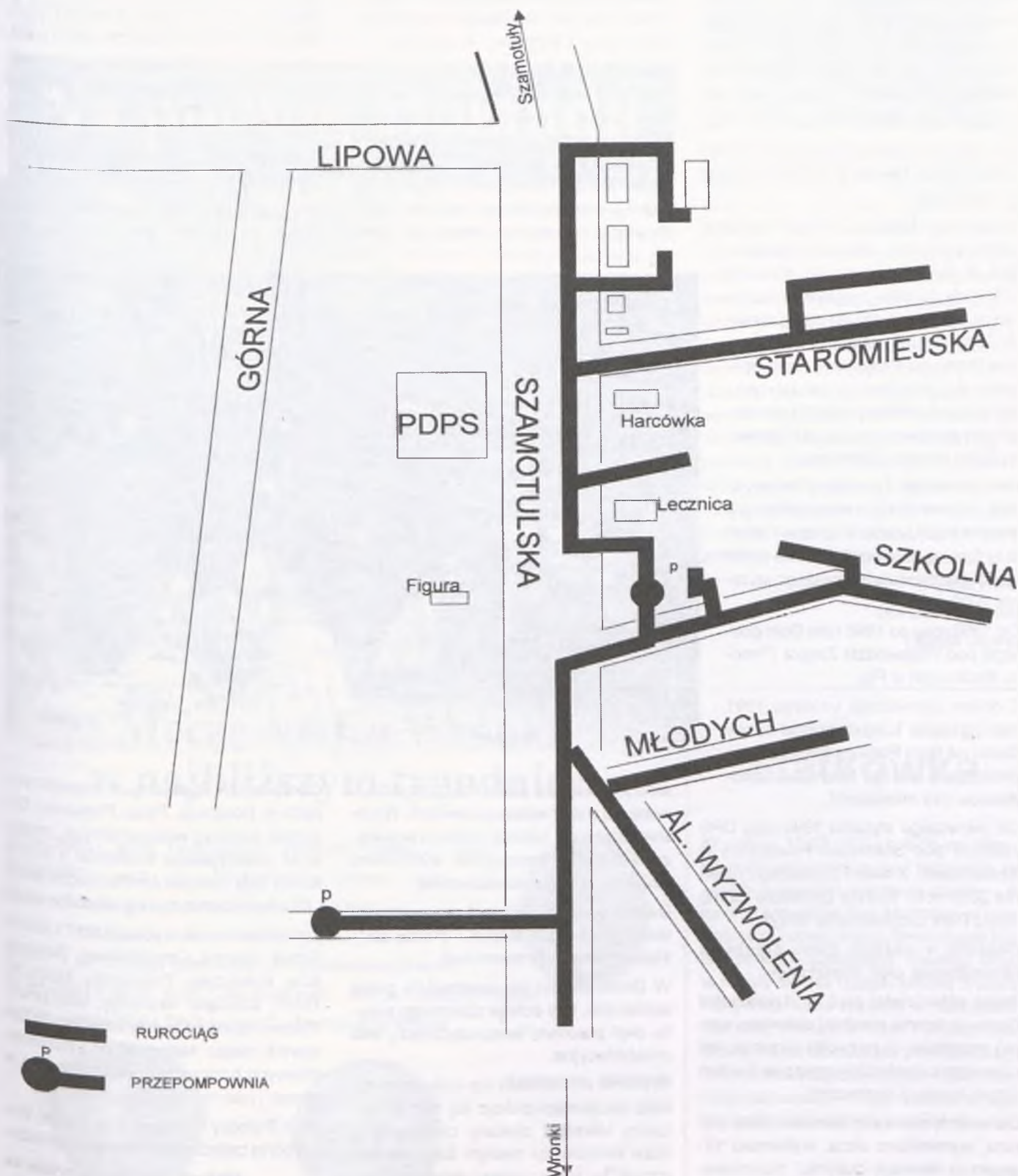
Nowa Wieś - projektowane kanały sanitarne
