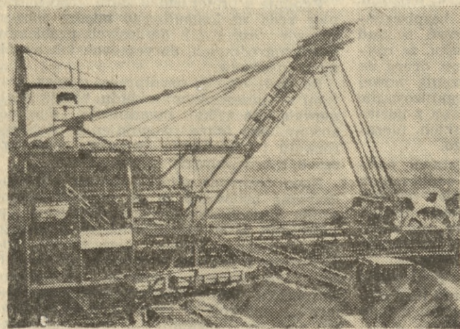
Na zdjęciu: W kopalni odkrywkowej „Freundschaft” w Klettwitz pracuje olbrzymia koparka „Sch RS 1000” wyprodukowana w Zakładach Budowy Maszyn „Lauchhammerwerk”. Koparka napędziana w ciągu 11 do 13 minut 8 specjalnych wagonów o pojemności 40 m³ każdy.
