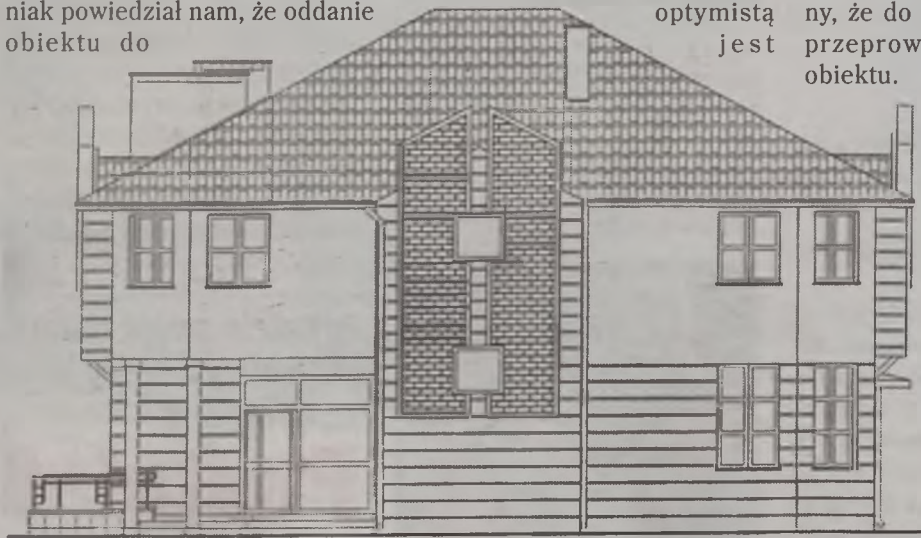
ELEVACJA FRONTOWA SKALA 1:100
