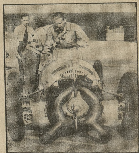
Samochód z motorem samolotowym, na którym hr. Trossi weźmie udział w wyścigach tegorocznych w Monzie. — Monstrum!
