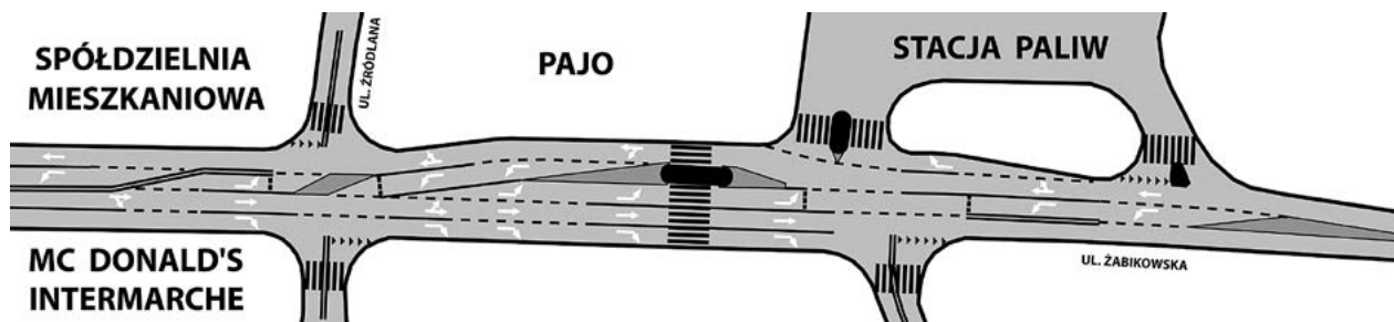
Organizacja ruchu drogowego na ul. Żabikowskiej, na odcinku pomiędzy ul. Powstańców Wlkp. a rondem Żabikowskim. Na czarno oznaczono wyspy, ciemno-szaro malowane obszary wyłączony z ruchu pojazdów rys. Rafał Wojtyniak
