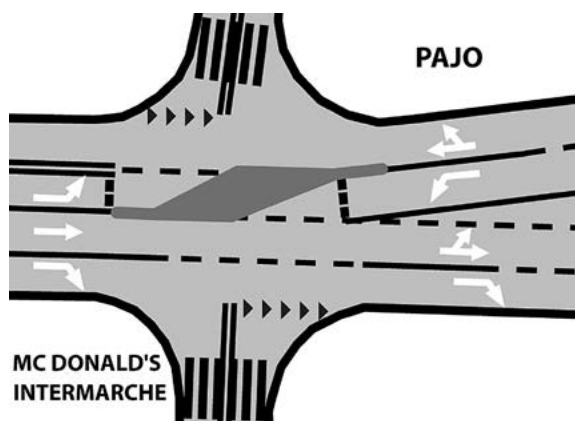
Organizacja ruchu drogowego na ul. Żabikowskiej, na odcinku pomiędzy ul. Powstańców Wlkp. a rondem Żabikowskim. Na czarno oznaczono wyspy, ciemno-szaro malowane obszary wyłączony z ruchu pojazdów rys. Rafał Wojtyniak
