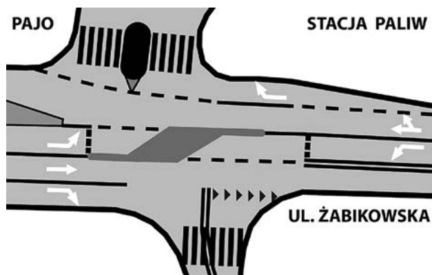
Skrzyżowanie Żabikowska-Paderewskiego. Proponowana wyspa z tworzywa sztucznego, mocowana do nawierzchni, wymuszająca wykonywanie prawidłowych manewrów rys. Rafał Wojtyniak
