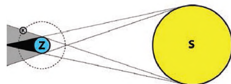
Schemat zaćmienia Księżyca – wzajemne ułożenie obiektów i istniejących cieni
