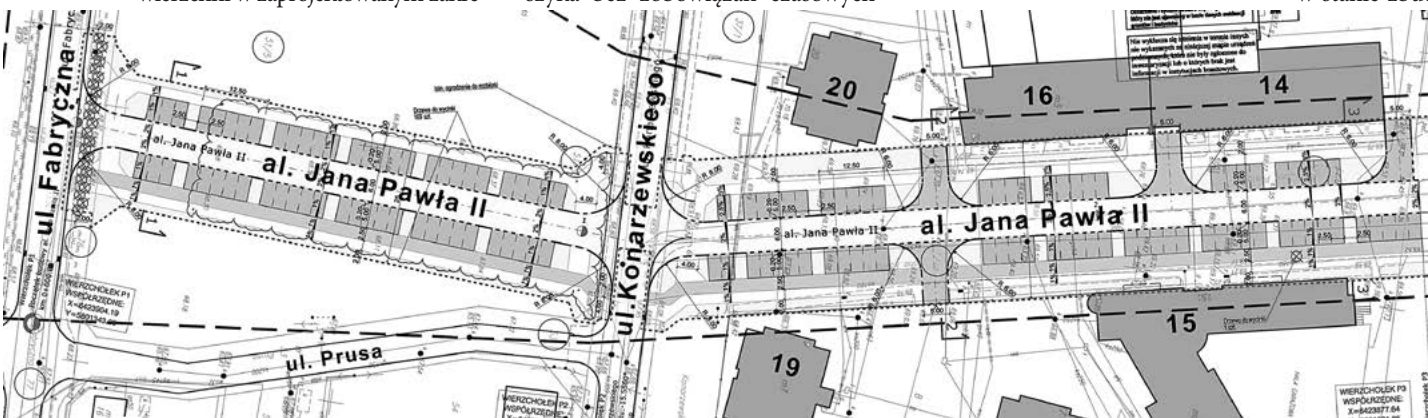
Projekt al. Jana Pawła II od ronda z ul. Wschodnią do ul. Fabrycznej. Nowy dukt pomiędzy ulicami Konarzewskiego a Fabryczną wytyczony tuż obok istniejącej ul. Prusa (w przyszłości ślepa – patrz fragment Miejscowego planu) oprac. SD Projekt s.c.
