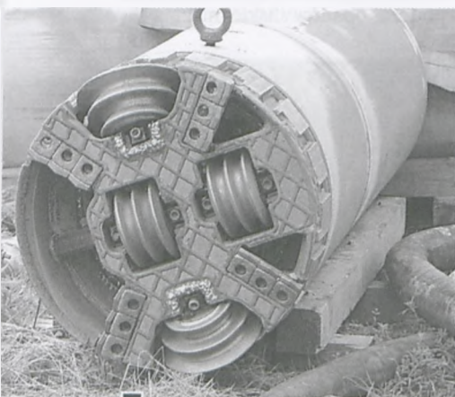
Specjalna głowica do frezowania gruntu metodą mikrotunelingu do wprowadzenia rur o średnicy 50 cm fot. Piotr P. Ruskowski
