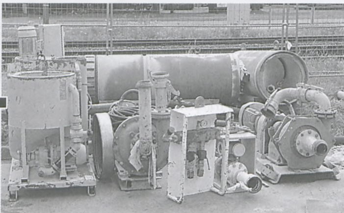
Zestaw urządzeń do mikrotunelingu fot. Piotr P. Ruskowski
