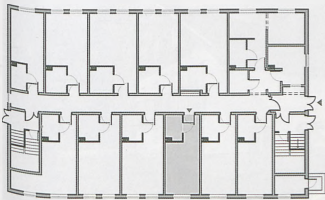
Rzut parteru pierwszego obiektu hotelowego z 51 mieszkaniami na 4 kondygnacjach www.grupa pajo
