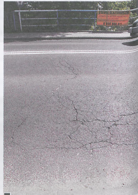
Spękana nawierzchnia jezdni na mostku na ul. Żabikowskiej mogą świadczyć o usterekach w konstrukcji fot. Michał Głazik
