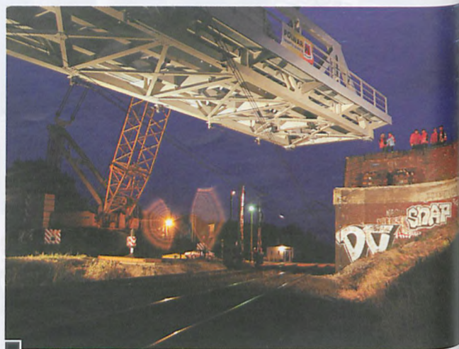
Osadzenie nowego przęsła unoszonego nad siecią trakcyjną za pomocą dwóch ciężkich dźwигów. Widok na południowy przyczółek wiaduktu i plac budowy w niedzielną noc. U dołu linia kolejowa Poznań-Wrocław fot. Przemysław Maćkowiak
